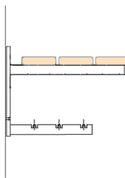
Modell 6220 Bankkonsole für Wandbefestigung, mit Schuhrost
